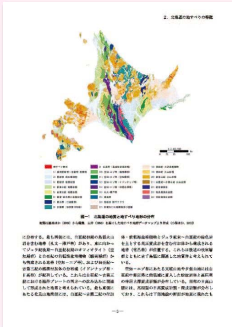
例：地すべりと地質との関係
